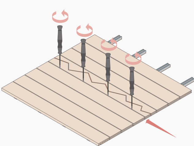
2. Desapretar CLIPS PRO · Unclipping CLIPS PRO · Déclipser CLIPS PRO · Расстегивание CLIPS PRO
