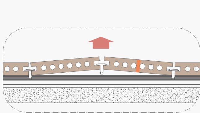
3. Retirar lama a sustituir · Remove slat to be replaced · Retirer la latte à remplacer · Снимите планку, которую необходимо заменить
