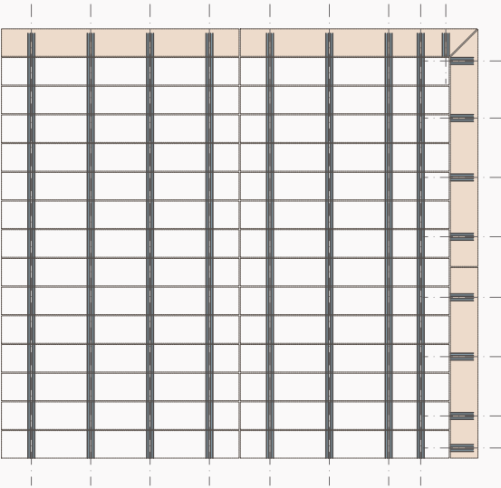
MONTAJE ALINEADO. Esquema en planta ALIGNED MOUNTING. Plan diagram · MONTAGE ALIGNÉ. Schéma du plan · ВЫРОВНЕННАЯ СБОРКА. План-схема
