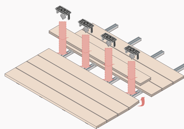
6. Montar base en CLIPS PRO + Nueva lama · Mount base on CLIPS PRO + New slat · Monter la base sur CLIPS PRO + Nouvelle lamelle · Монтируйте основание на CLIPS PRO + Новая планка
