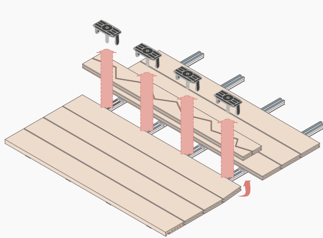
4. Retirar CLIPS PRO · Remove CLIPS PRO · Retirer les CLIPS PRO · Отозвать CLIPS PRO
