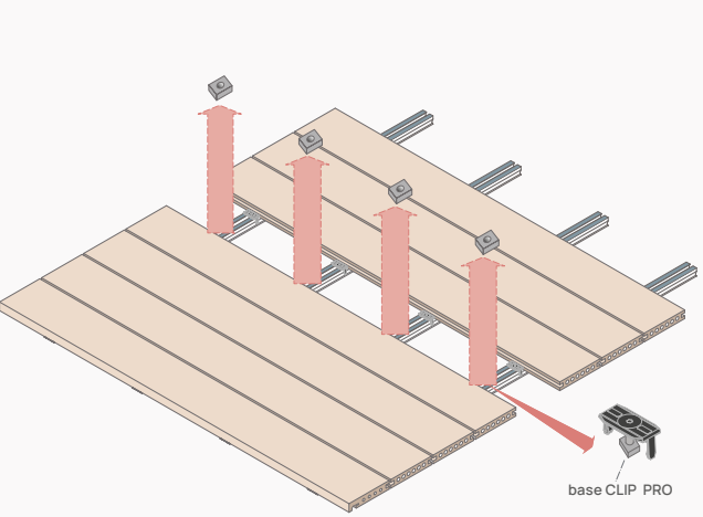
5. Retirar bases CLIPS PRO · Remove CLIPS PRO bases · Retirer les bases CLIPS PRO · Удалите основания CLIPS PRO
